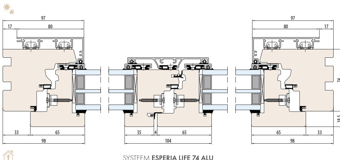
SYSTEEM ESPERIA LIFE 74 ALU wisselstijl (horizontale doorsnede)
