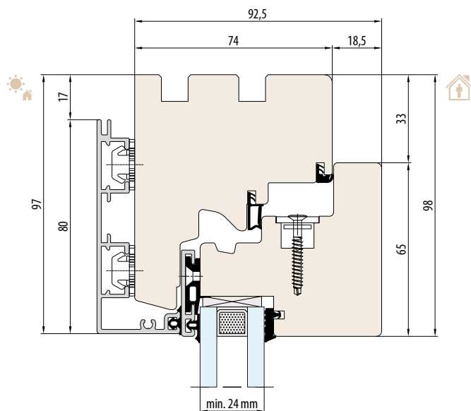
VERTICALE DOORSNEDE A-A
