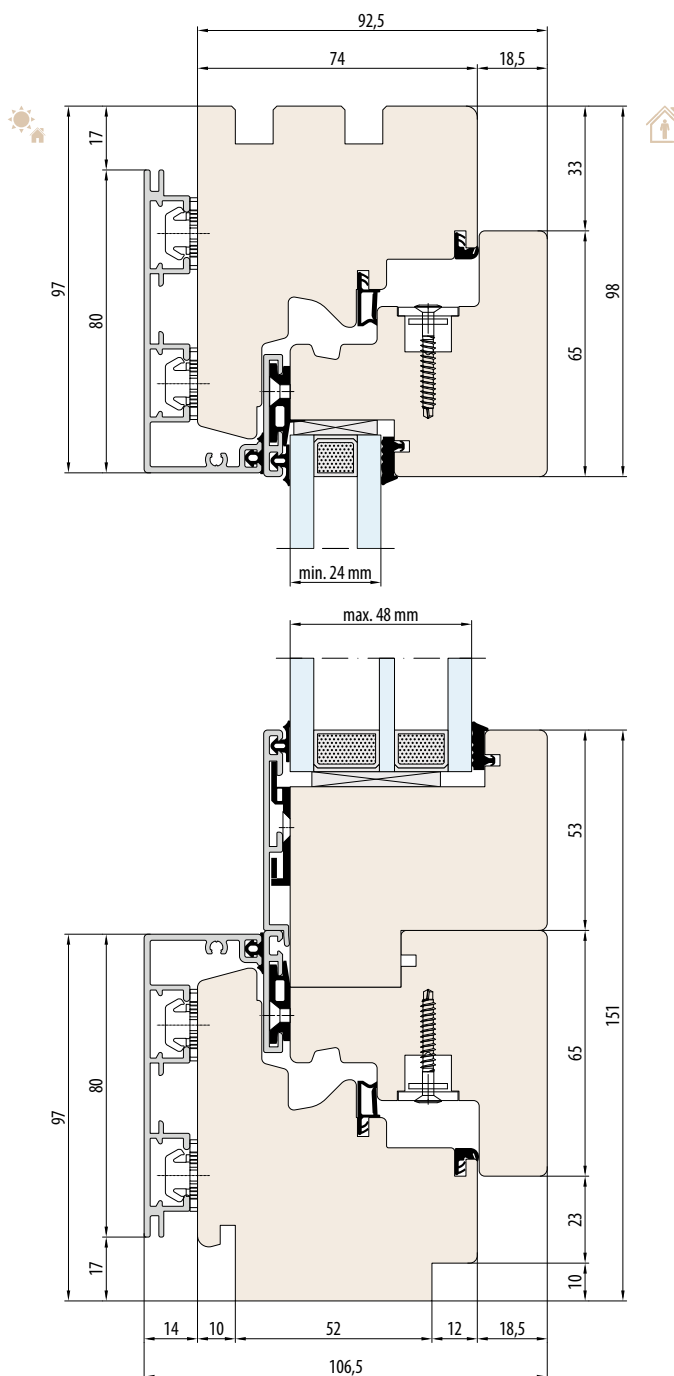
SYSTEEM ESPERIA LIFE 74 ALU enkelvleugelige balkondeuren met hoge drempel
