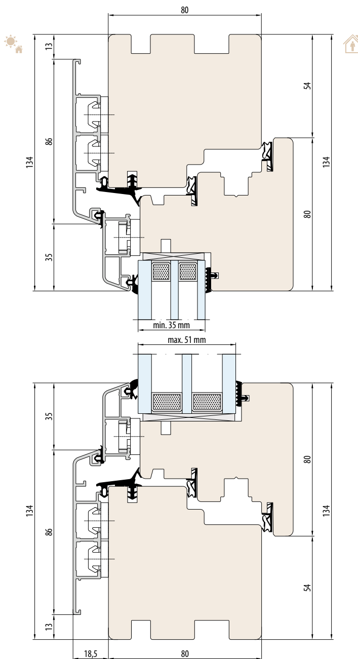
SYSTEEM NATURO 80 ALU GEMINI CLASSIC zonder sponning voor vensterbank
