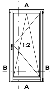
VERTICALE DOORSNEDE A-A
