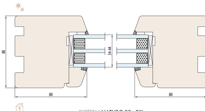
SYSTEEM NATURO 80 - FIX horizontale doorsnede
