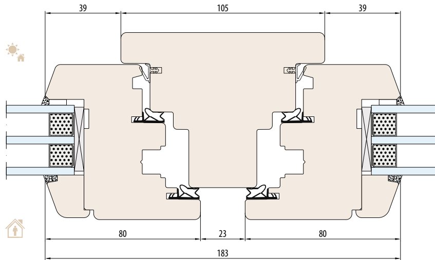
SYSTEEM NATURO 80 vaste stijl 105 mm
