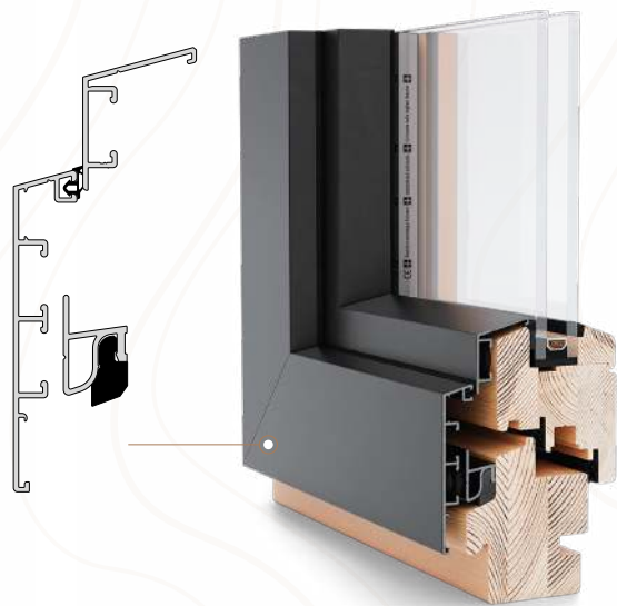
Profil Reno Line (met sponning)
