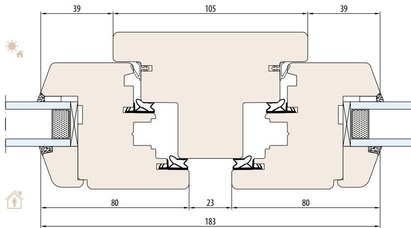
SYSTEEM NATURO 68 vaste stijl 105 mm
