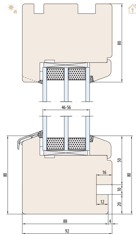
SYSTEEM NATURO 92 - FIX spionning voor vensterbank intern
