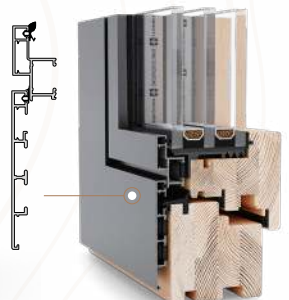
GEMINI QUADRAT FB Standaard profiel (zonder sponning)
