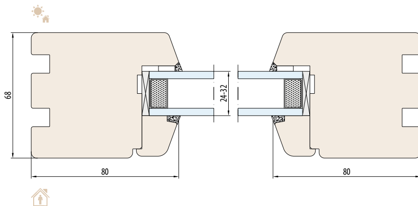
SYSTEEM NATURO 68 - FIX horizontale doorsnede
