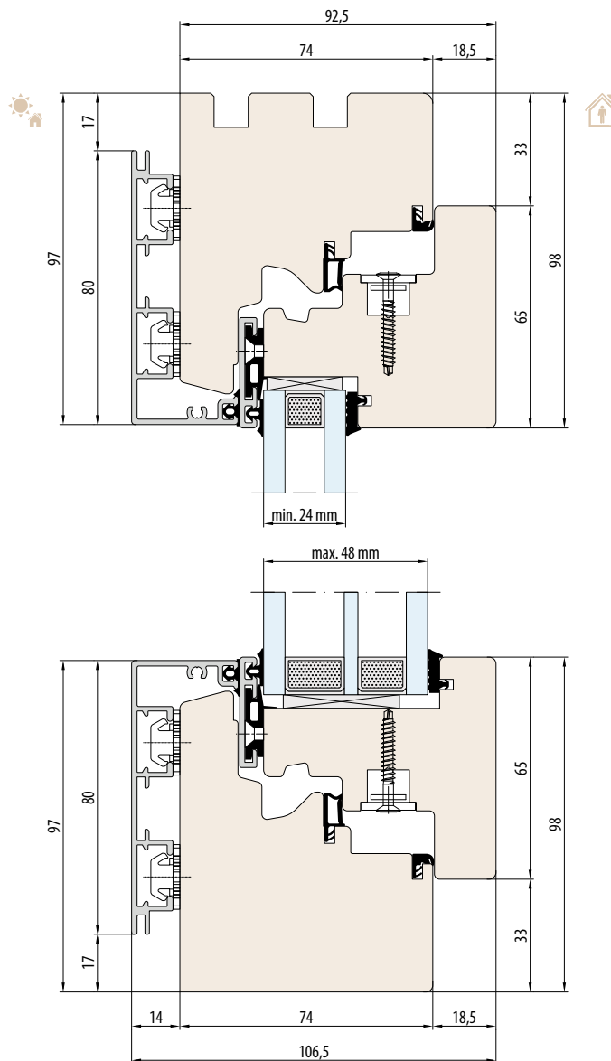
SYSTEEM ESPERIA LIFE 74 ALU zonder sponning voor vensterbank
