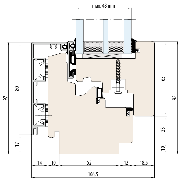
SYSTEEM ESPERIA LIFE 74 ALU sponing voor vensterbank intern en extern
