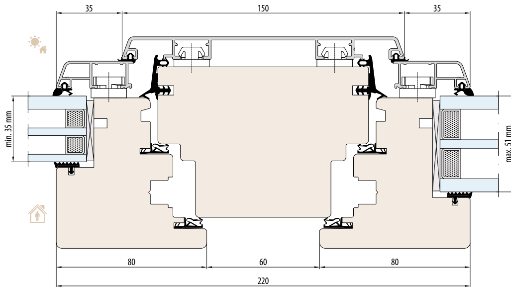
SYSTEEM NATURO 80 ALU
