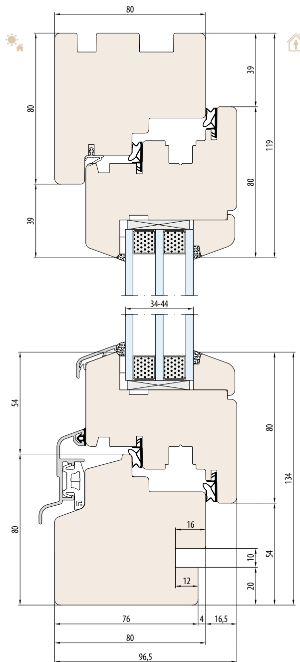
SYSTEEM NATURO 80 sponning voor vensterbank intern
