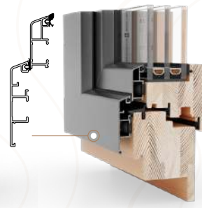
GEMINI CLASSIC Renovatieprofiel (met sponning)
