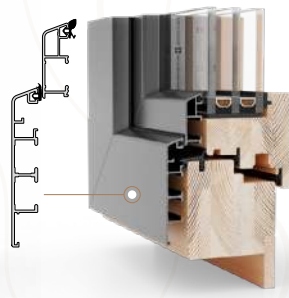
GEMINI CLASSIC Renovatieprofiel (zonder sponning)
