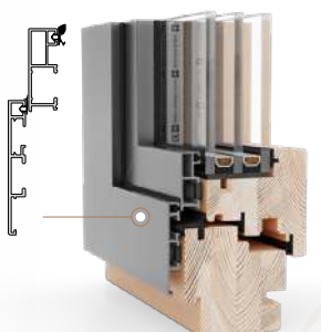
GEMINI QUADRAT Standaard profiel (met sponning)
