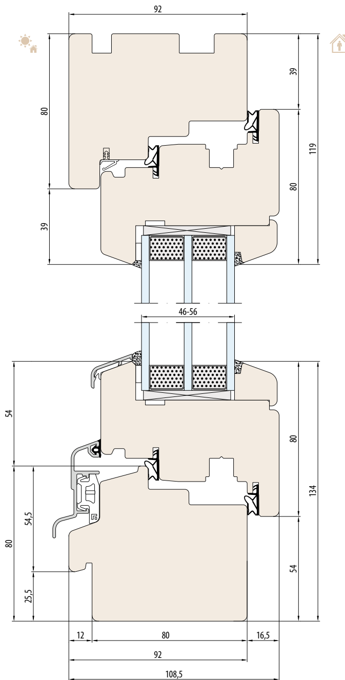
SYSTEEM NATURO 92 spinning voor vensterbank extern
