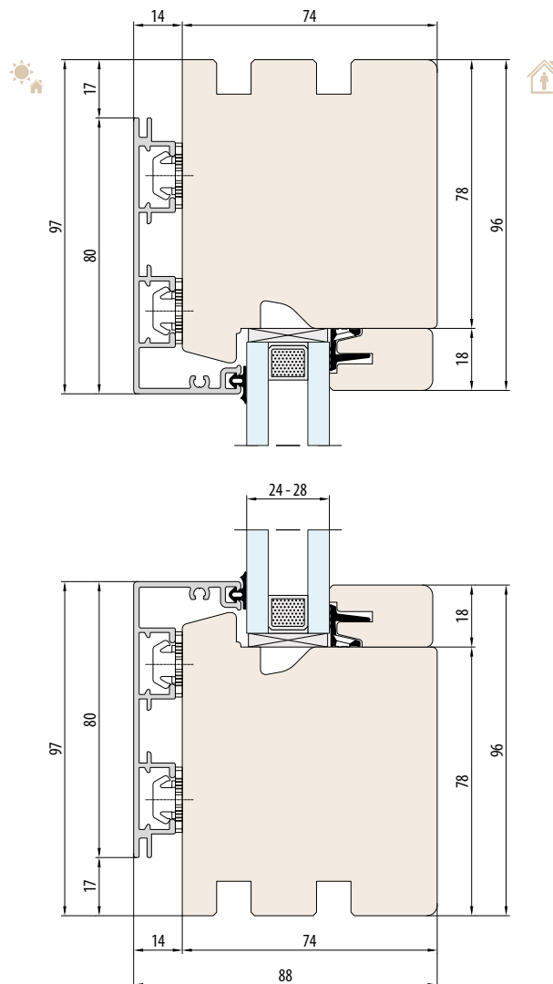
SYSTEEM ESPERIA LIFE 74 ALU - FIX zonder sponning voor vensterbank
