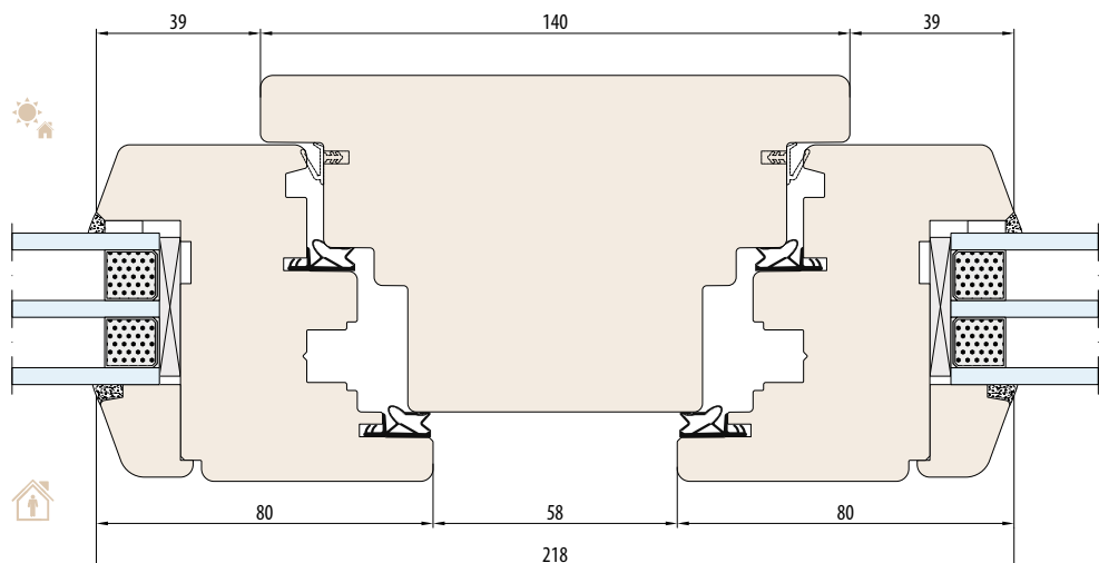
SYSTEEM NATURO 80 vaste stijl 140 mm
