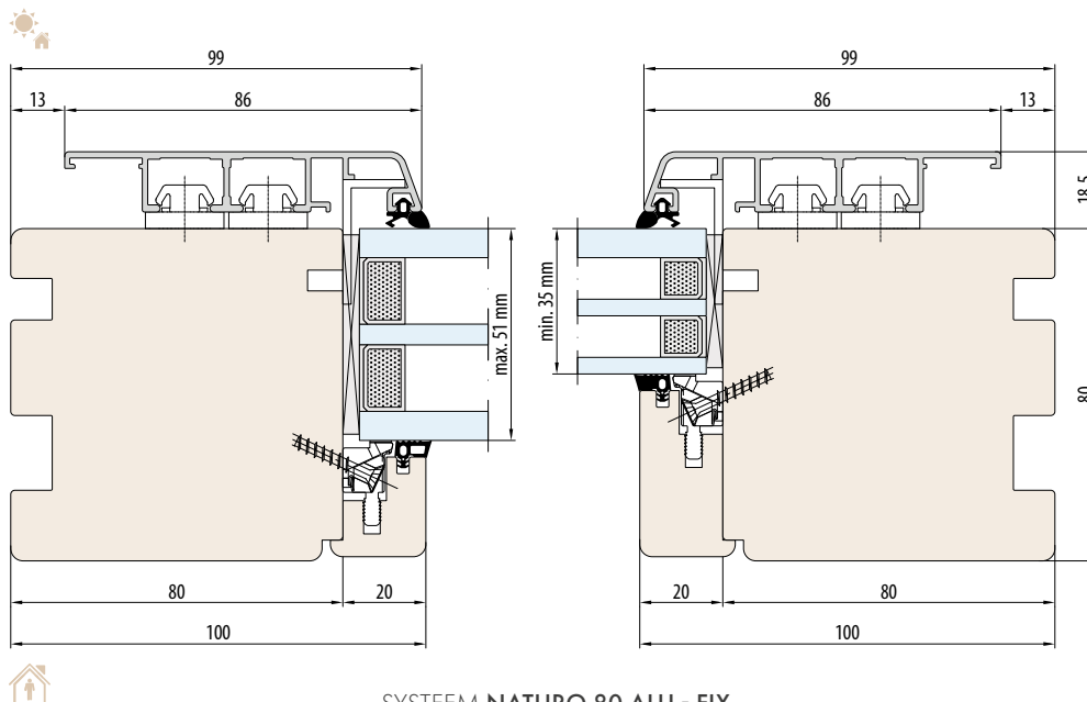
SYSTEEM NATURO 80 ALU - FIX
