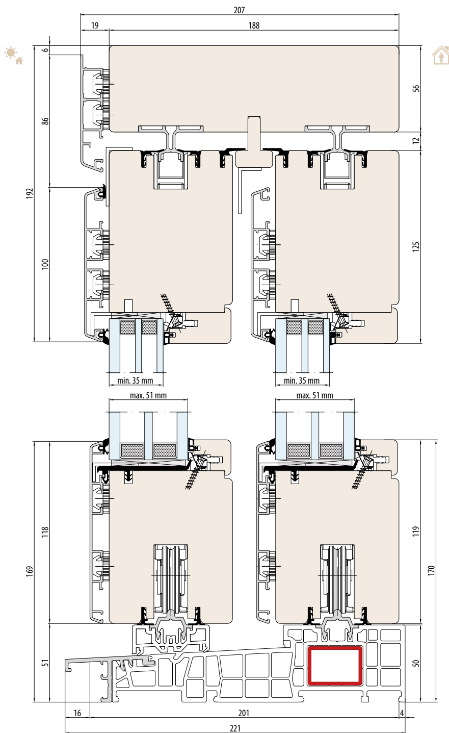
NATURO 80 HST ALU-SYSTEEM (algemene afmetingen) - drempel 50 mm - schema "D"
