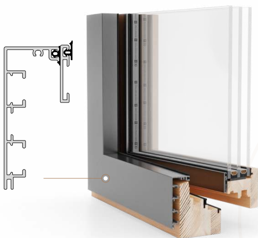
Standaard profiel (zonder sponning)
