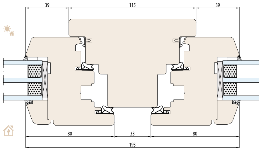
SYSTEEM NATURO 80 vaste stijl 115 mm
