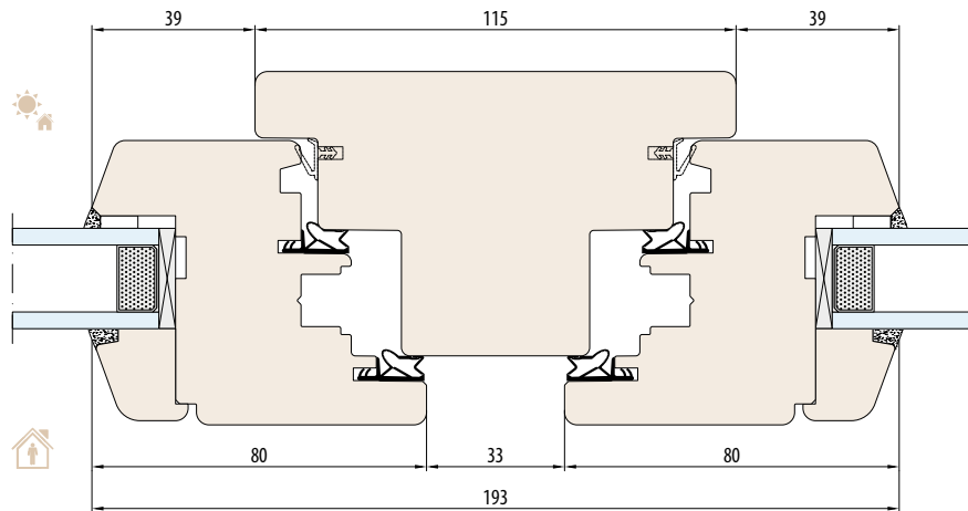
SYSTEEM NATURO 68 vaste stijl 115 mm
