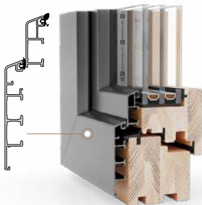
GEMINI CLASSIC Standaard profiel (zonder sponning)
