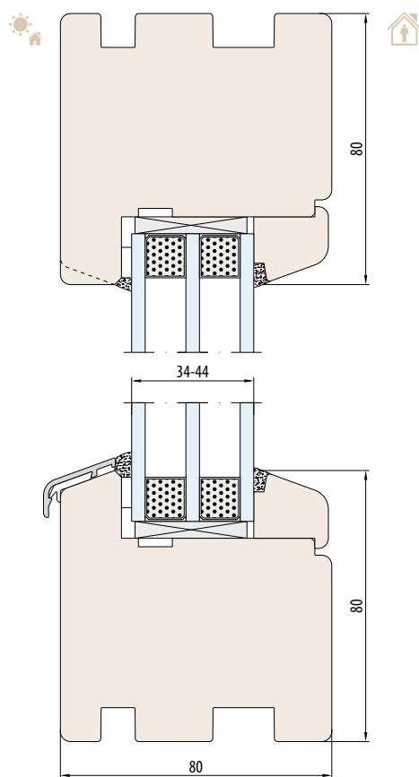
SYSTEEM NATURO 80 - FIX zonder sponning voor vensterbank
