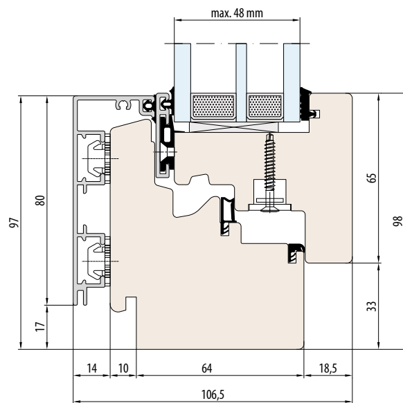
SYSTEEM ESPERIA LIFE 74 ALU sponing voor vensterbank extern
