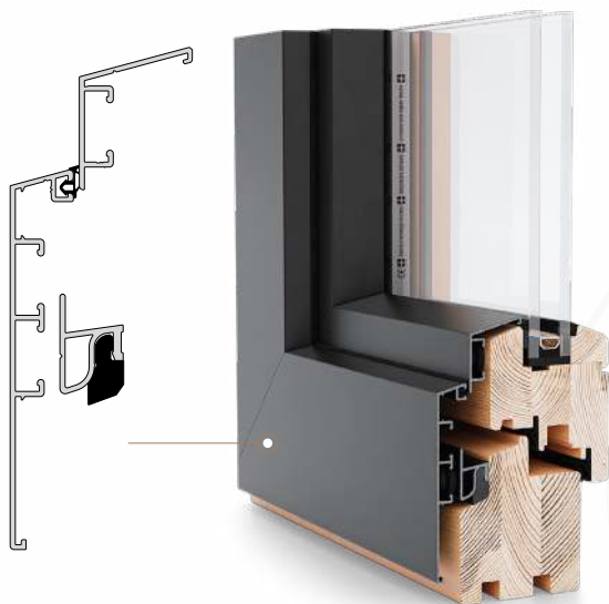
Profil Reno Line (zonder sponning)
