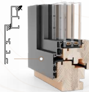
MIRA CONTOUR Standaard profiel (met sponning)
