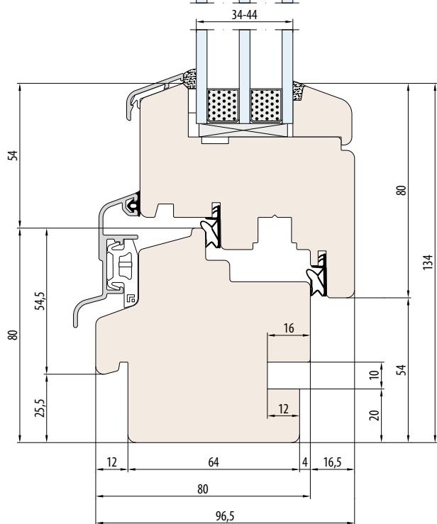
SYSTEEM NATURO 80 sponning voor vensterbank intern en extern
