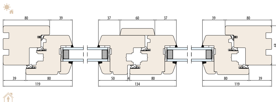
SYSTEEM NATURO 68 wisselstijl (horizontale doorsnede)
