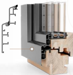
GEMINI CLASSIC Standaard profiel (met sponning)
