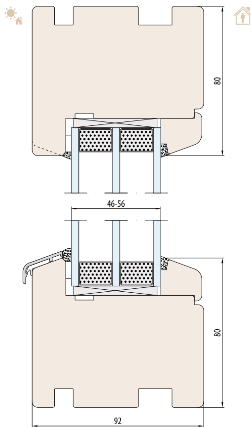
SYSTEEM NATURO 92 - FIX zonder sponning voor vensterbank
