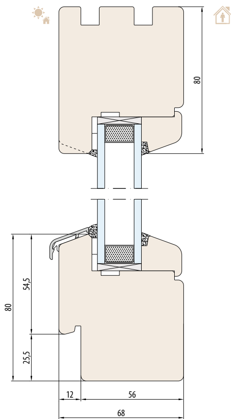
SYSTEEM NATURO 68 - FIX sponning voor vensterbank extern
