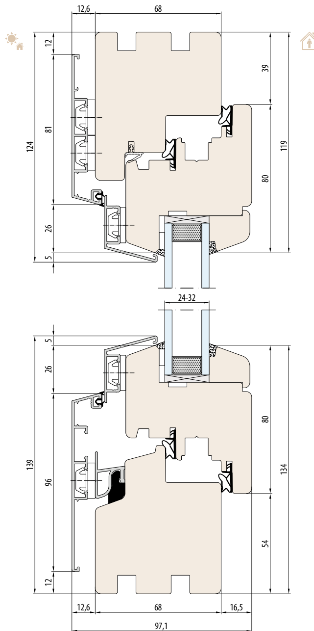
SYSTEEM NATURO 68 ALU RENO LINE zonder sponning voor vensterbank
