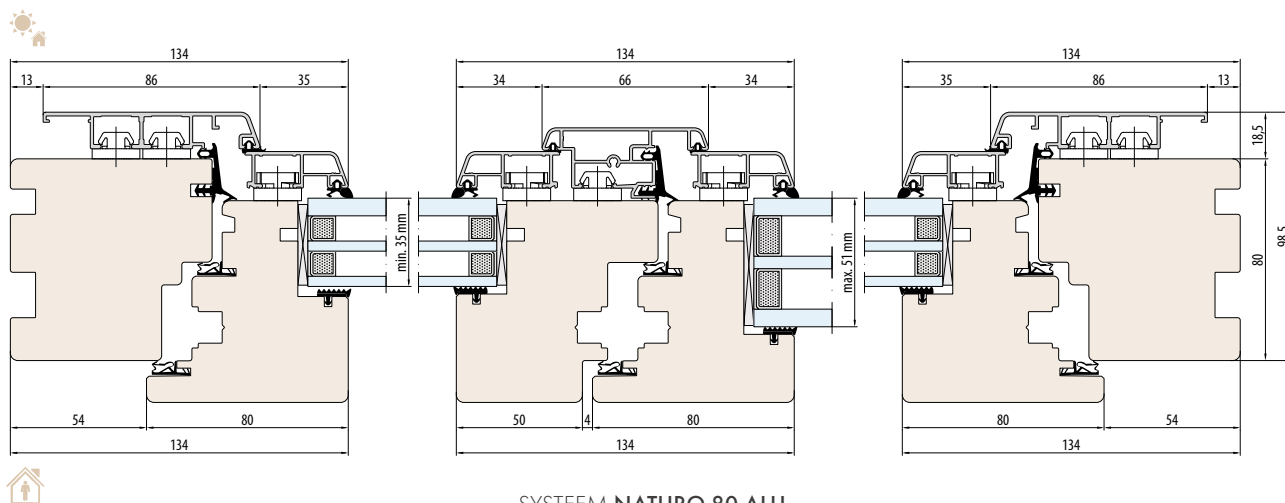
SYSTEEM NATURO 80 ALU
