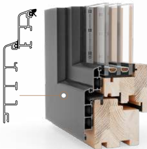
MIRA Standaard profiel (zonder sponning)
