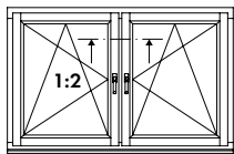
HORizontale DoorsneDe
