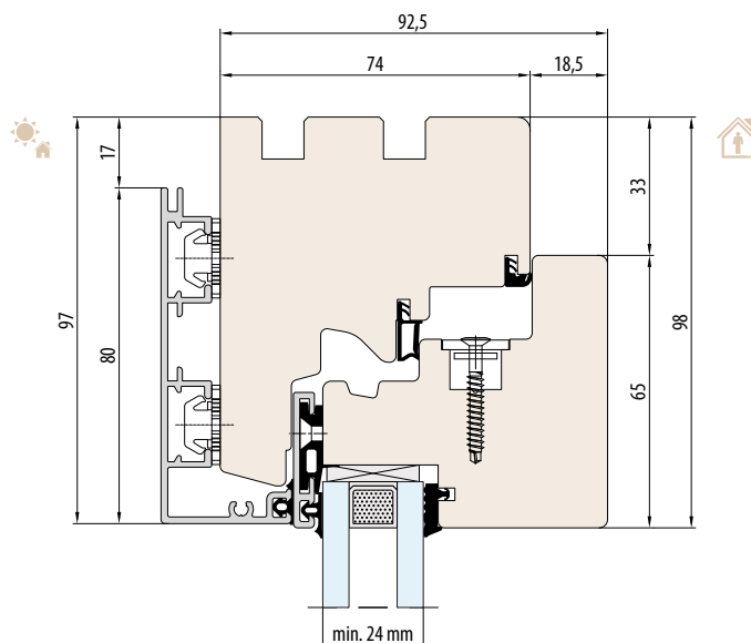
VERTICALE DOORSNEDE A-A
