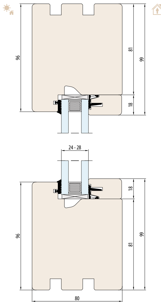
SYSTEEM ESPERIA LIFE 80 - FIX zonder sponning voor vensterbank
