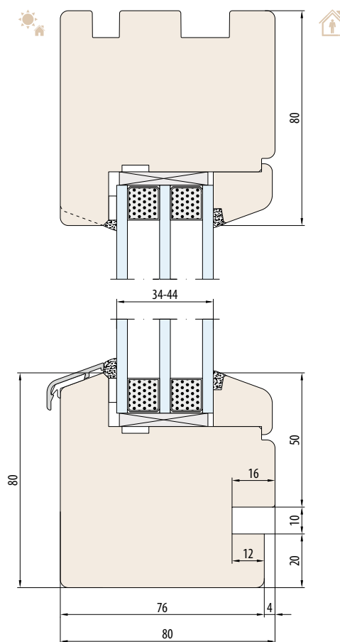
SYSTEEM NATURO 80 - FIX spinning voor vensterbank intern
