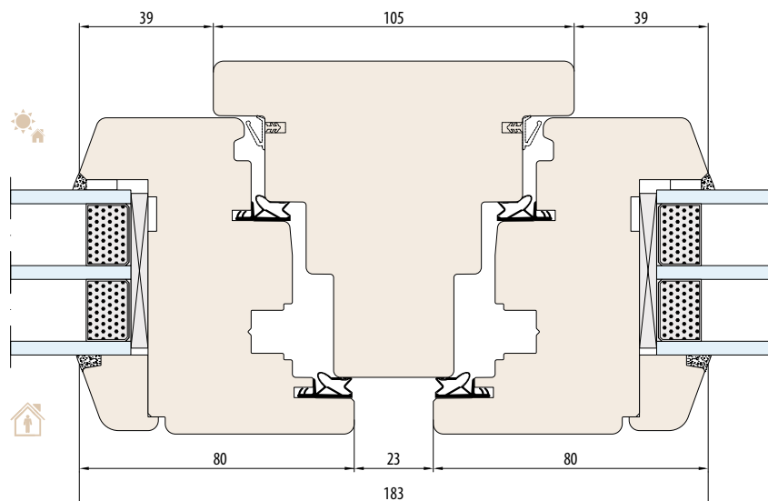
SYSTEEM NATURO 92 vaste stijl 105 mm
