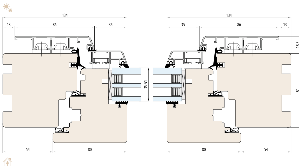
SYSTEEM NATURO 80 ALU GEMINI CLASSIC horizontale doorsnede
