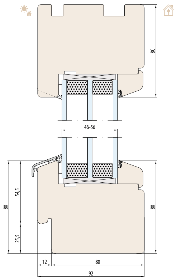
SYSTEEM NATURO 92 - FIX spionning voor vensterbank extern
