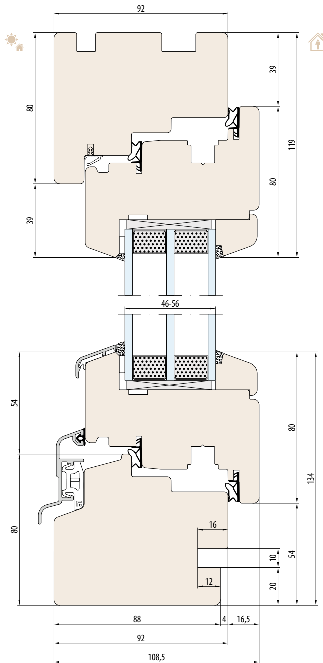
SYSTEEM NATURO 92 spinning voor vensterbank intern
