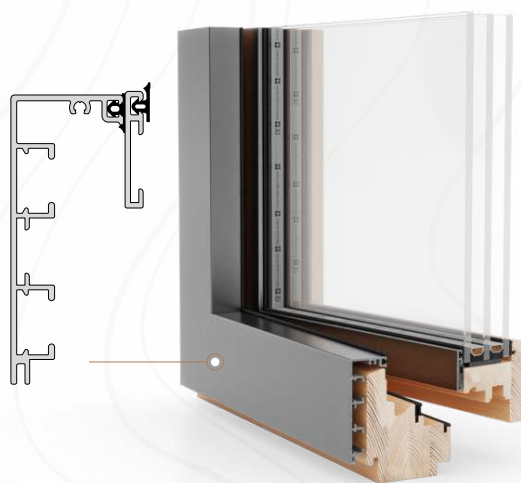
Standaard profiel (met sponning)
