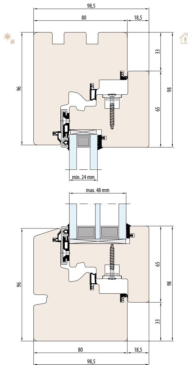
SYSTEEM ESPERIA LIFE 80 zonder sponning voor vensterbank
