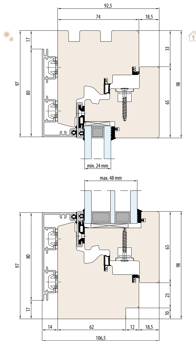
SYSTEEM ESPERIA LIFE 74 ALU spionning voor vensterbank intern
