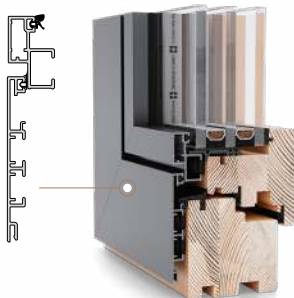
MIRA CONTOUR FB Standaard profiel (zonder sponning)
