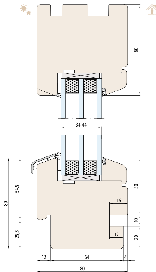
SYSTEEM NATURO 80 - FIX sponning voor vensterbank intern en extern
