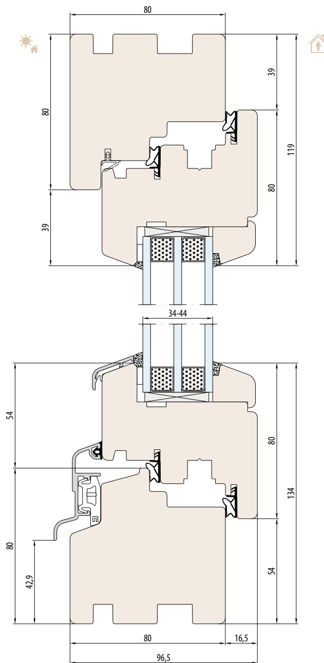
SYSTEEM NATURO 80 zonder sponning voor vensterbank
