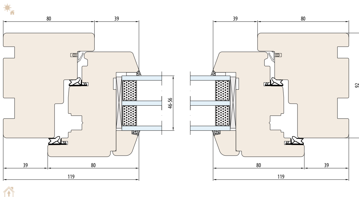
SYSTEEM NATURO 92 horizontale doorsnede
