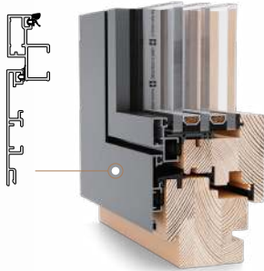
MIRA CONTOUR FB Standaard profiel (met sponning)
