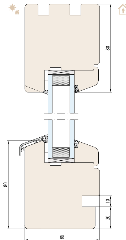
SYSTEEM NATURO 68 - FIX sponning voor vensterbank intern
