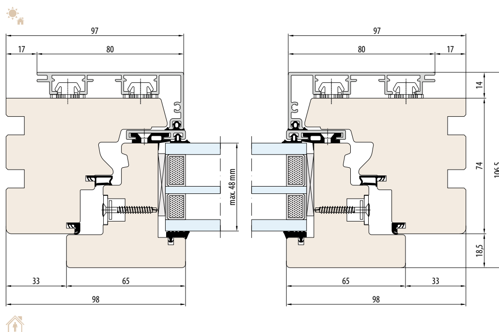
SYSTEEM ESPERIA LIFE 74 ALU horizontale doorsnede
