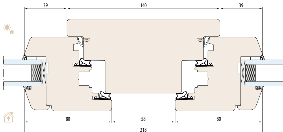
SYSTEEM NATURO 68 vaste stijl 140 mm
