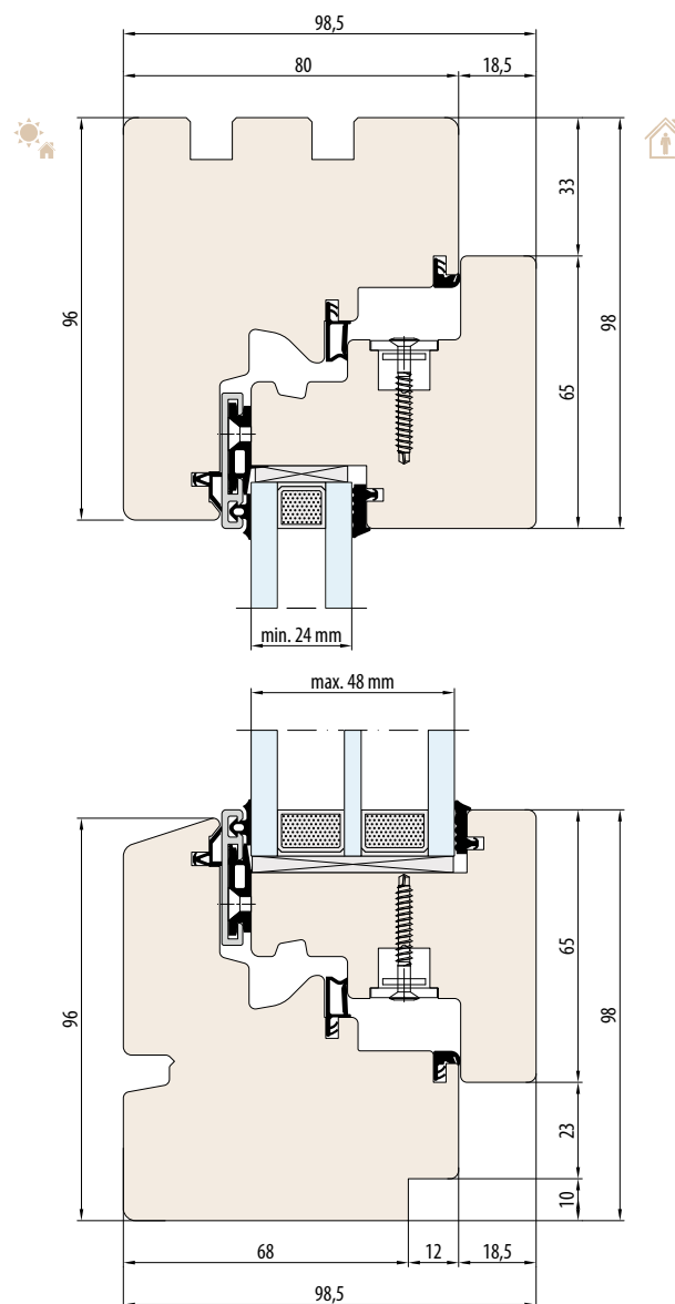
SYSTEEM ESPERIA LIFE 80 spionning voor vensterbank intern
