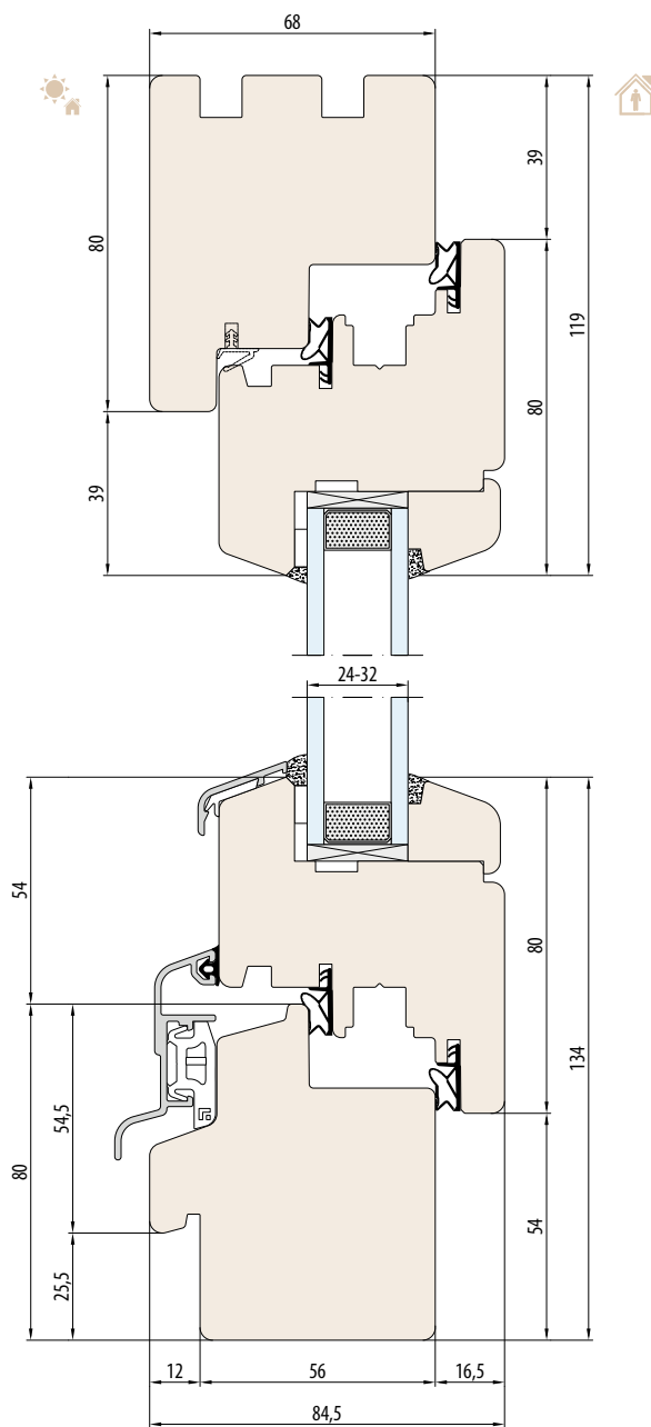
SYSTEEM NATURO 68 sponing voor vensterbank extern
