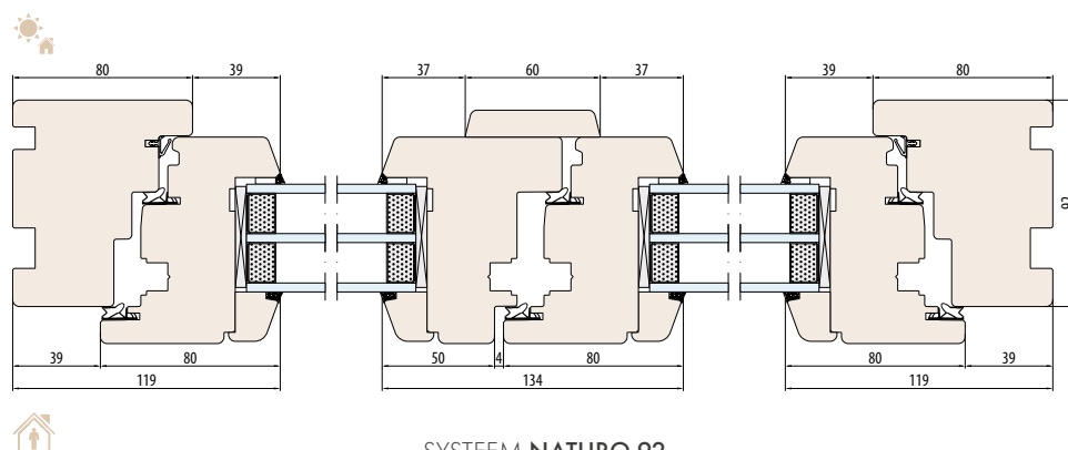
SYSTEEM NATURO 92 wisselstijl (horizontale doorsnede)
