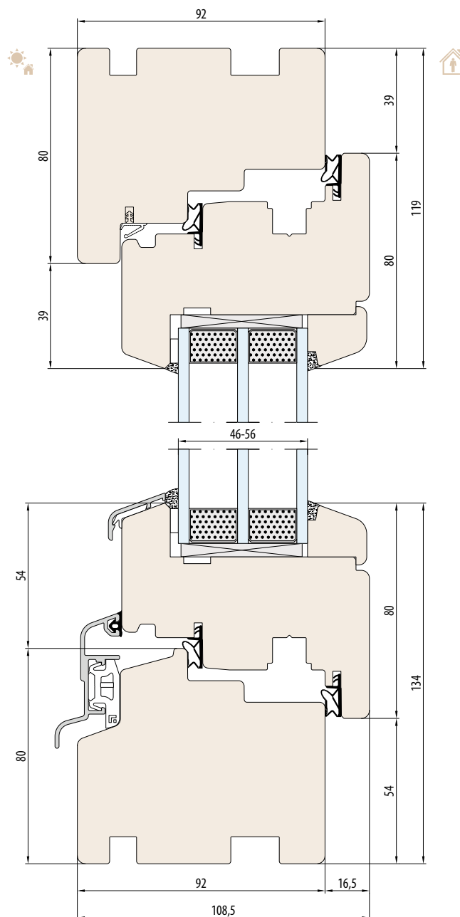
SYSTEEM NATURO 92 zonder sponning voor vensterbank
