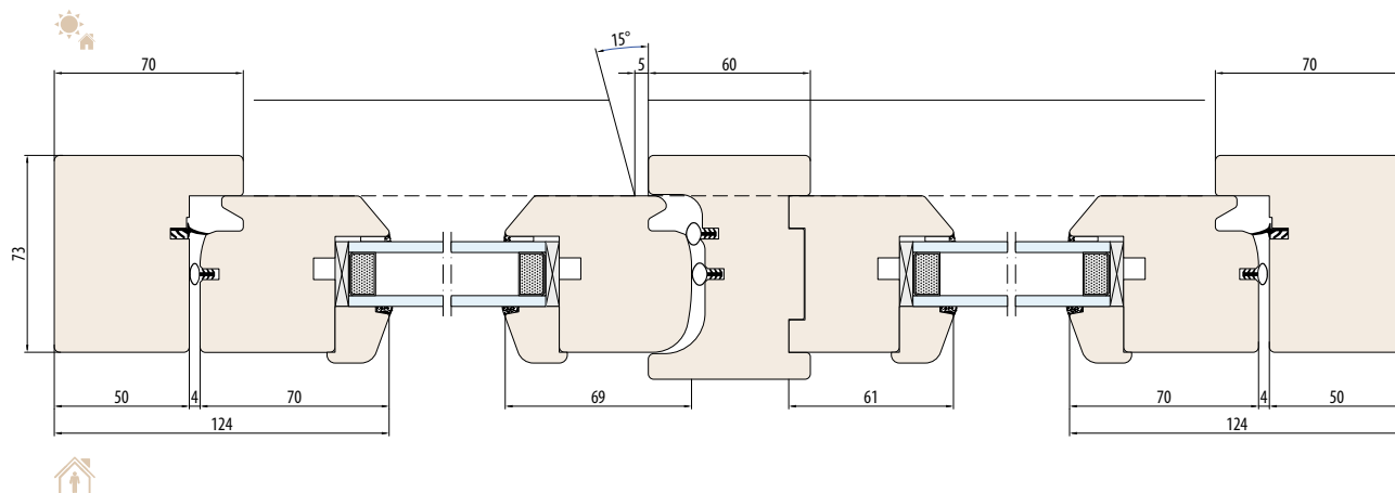
GUEULE DE LOUP-SYSTEEM draaistijl, stijl - horizontale doorsnede
