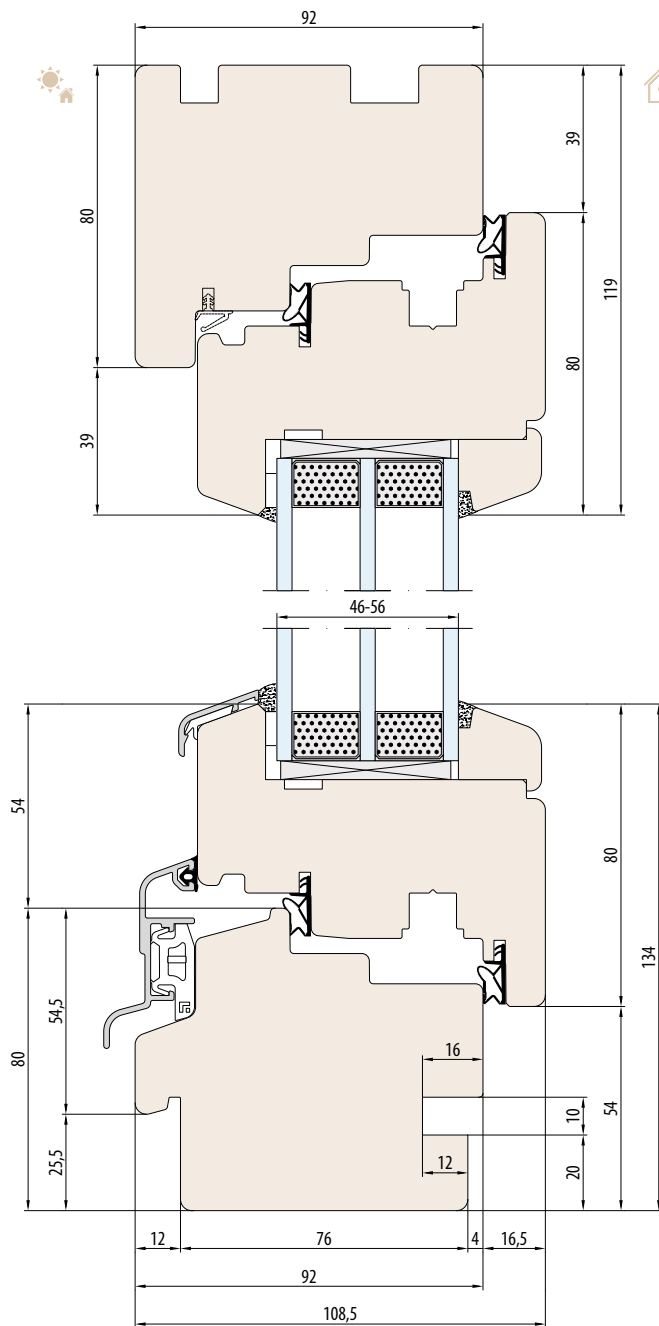
SYSTEEM NATURO 92 spinning voor vensterbank intern en extern
