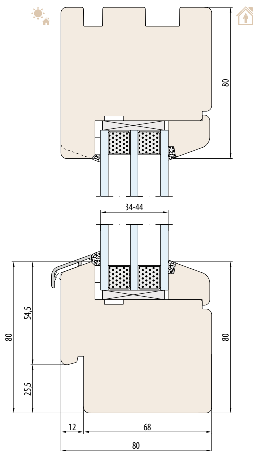
SYSTEEM NATURO 80 - FIX spinning voor vensterbank extern
