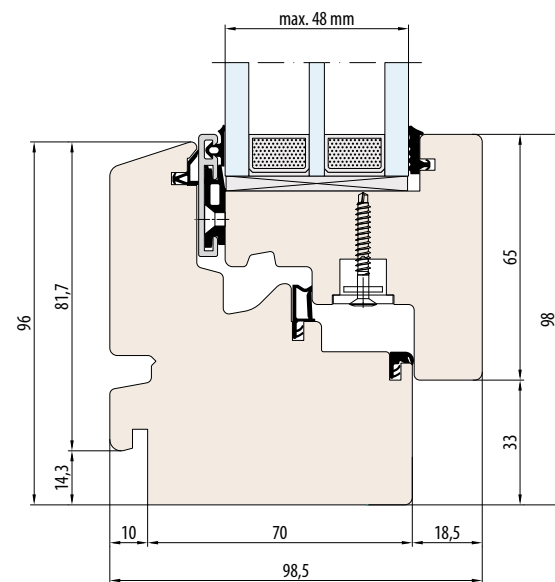
SYSTEEM ESPERIA LIFE 80 sponning voor vensterbank extern
