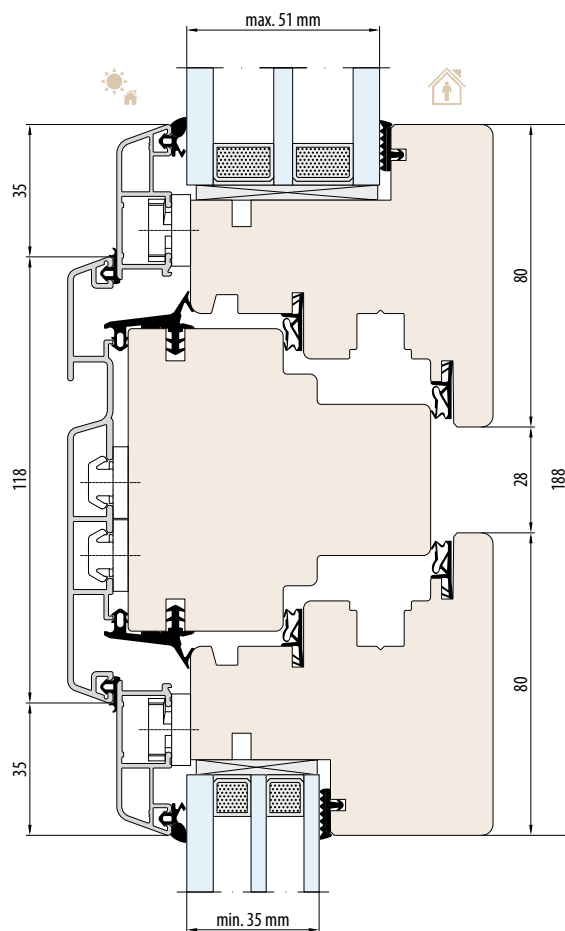
SYSTEM NATURO 80 ALU GEMINI CLASSIC tussendorpel 80 mm
