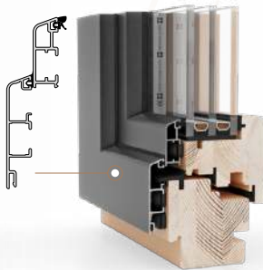
MIRA Standaard profiel (met sponning)
