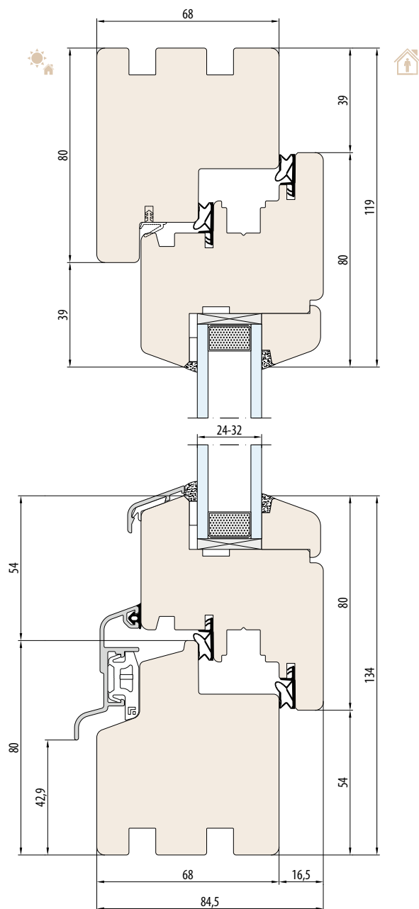
SYSTEEM NATURO 68 zonder sponning voor vensterbank
