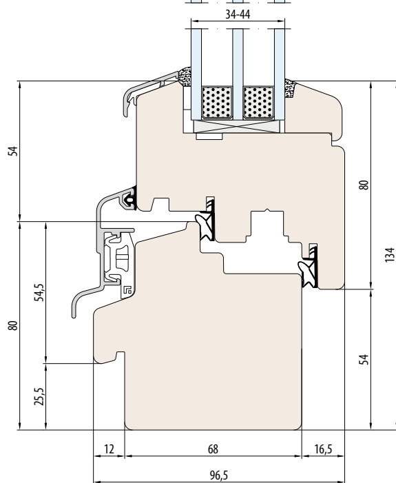
SYSTEEM NATURO 80 sponning voor vensterbank extern
