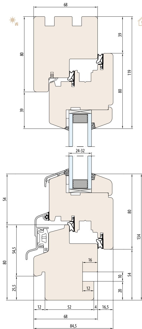
SYSTEEM NATURO 68 sponing voor vensterbank intern en extern
