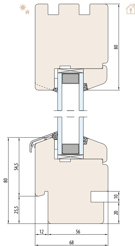
SYSTEEM NATURO 68 - FIX sponning voor vensterbank intern en extern
