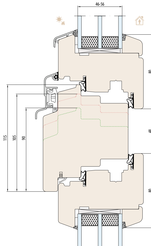
SYSTEEM NATURO 92 tussendorpel: 90 mm, 105 mm, 115 mm
