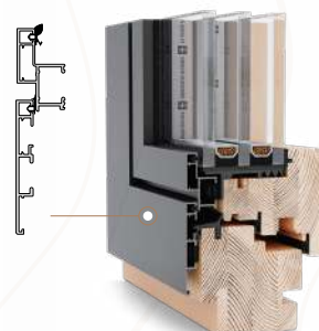
GEMINI QUADRAT FB Standaard profiel (met sponning)
