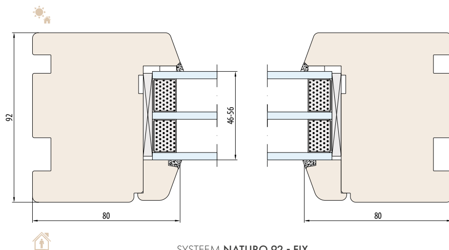
SYSTEEM NATURO 92 - FIX horizontale doorsnede
