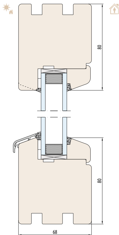
SYSTEEM NATURO 68 - FIX zonder sponning voor vensterbank
