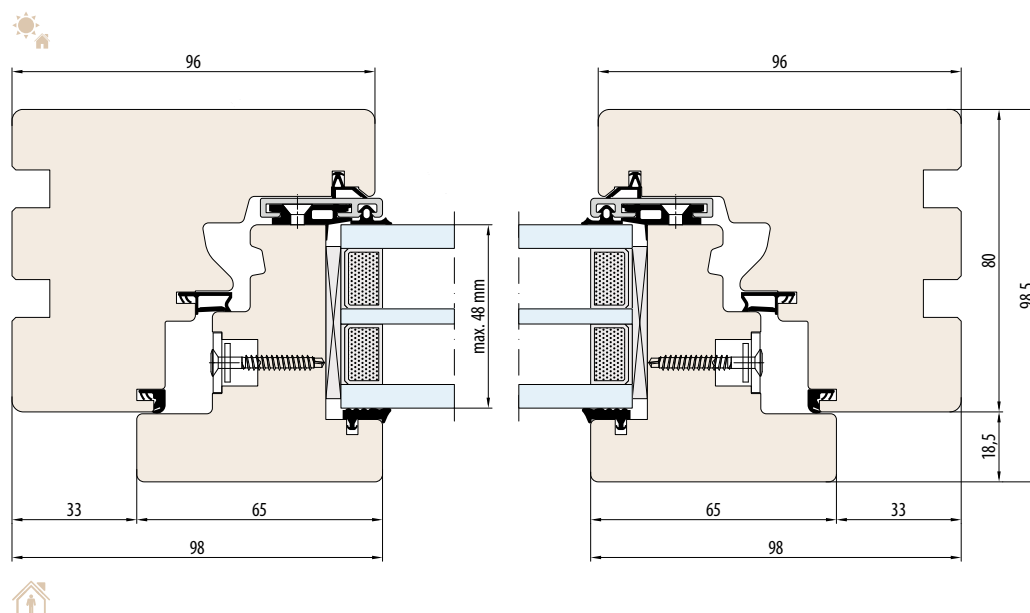
SYSTEEM ESPERIA LIFE 80 horizontale doorsnede
