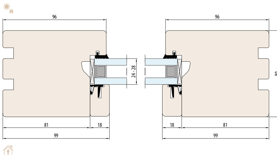
SYSTEEM ESPERIA LIFE 80 - FIX horizontale doorsnede
