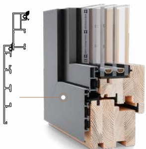
GEMINI QUADRAT Standaard profiel (zonder sponning)
