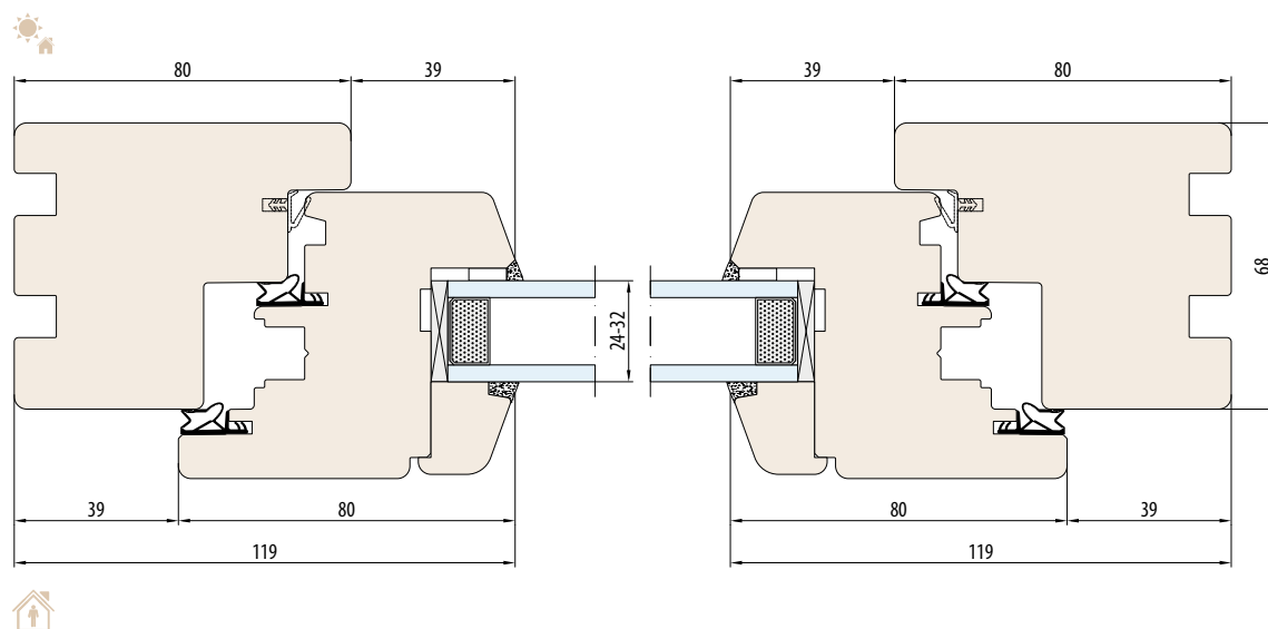
SYSTEEM NATURO 68 horizontale doorsnede
