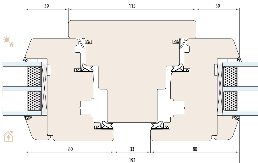
SYSTEEM NATURO 92 vaste stijl 115 mm
