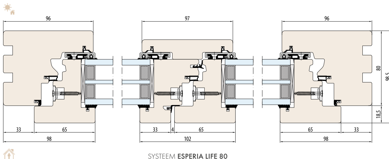
SYSTEEM ESPERIA LIFE 80 wisselstijl (horizontale doorsnede)
