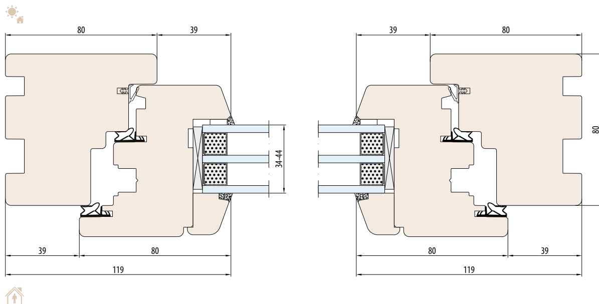
SYSTEEM NATURO 80 horizontale doorsnede
