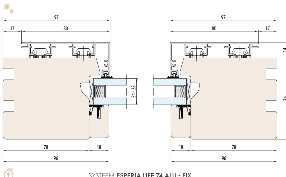
SYSTEEM ESPERIA LIFE 74 ALU - FIX horizontale doorsnede
