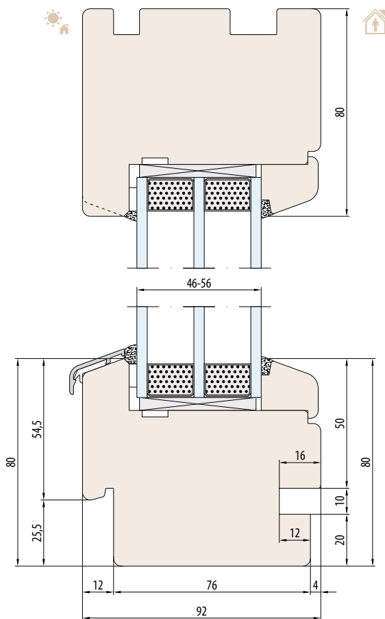
SYSTEEM NATURO 92 - FIX sponning voor vensterbank intern en extern
