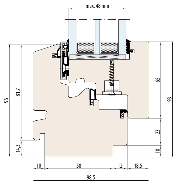
SYSTEEM ESPERIA LIFE 80 sponning voor vensterbank intern en extern
