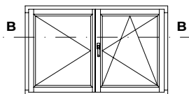
HORizontALE DOORSNEDE B-B
