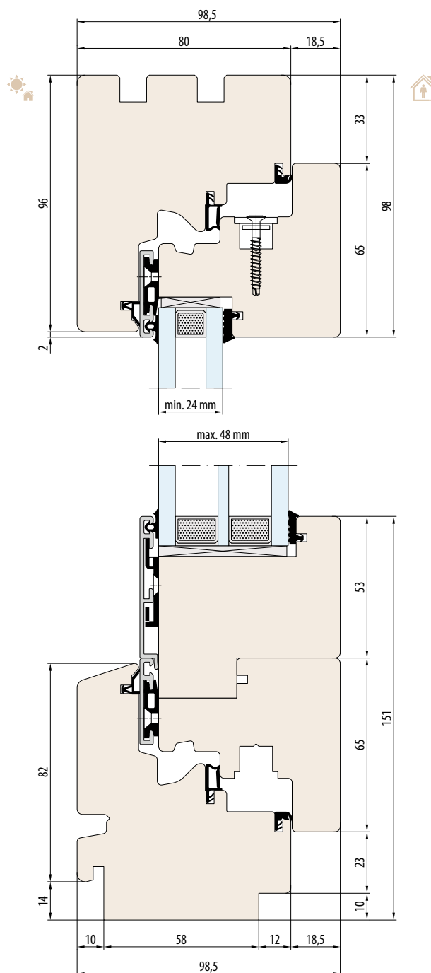
SYSTEEM ESPERIA LIFE 80 enkelvleugelige balkondeuren met hoge drempel
